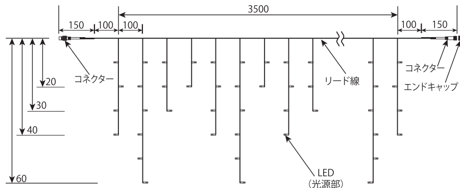
LED 色 : 黄 品番 : T-100V-CB-VCJ-CPY
