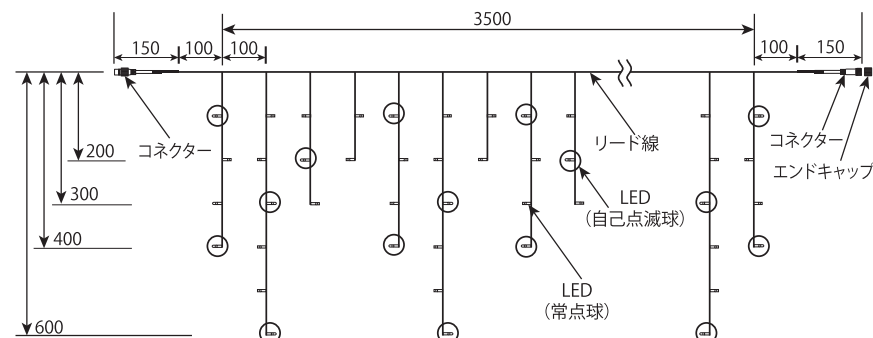
LED 色 : 黄 品番 : T-100V-CB-VHT-CPY
