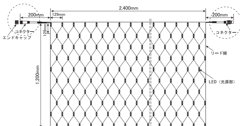
LED 色 : 黄 品番 : N-100V-BB-VCJ-CPY
