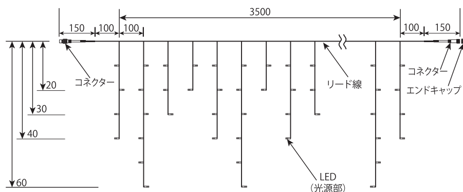
LED 色 : 黄 品番 : T-100V-BB-VCJ-CPY
